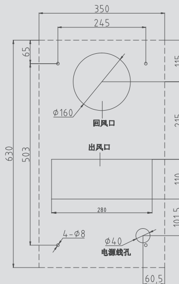
KT600开孔图 KT600 portiforium drawing
