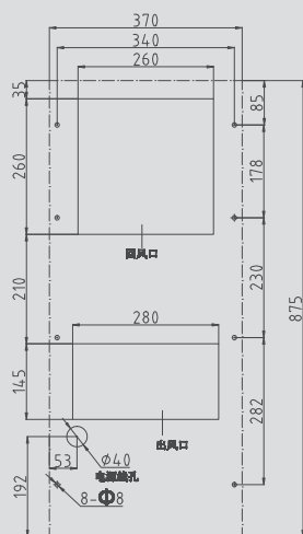
KT1500开孔图 KT1500 portiforium drawing
