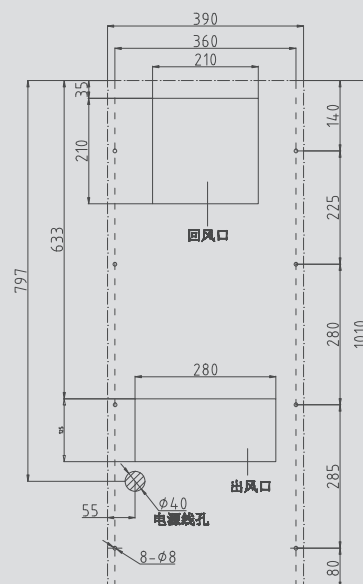
KT2000开孔图 KT2000 portiforium drawing
