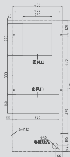
KT3200开孔图 KT3200 portiforium drawing
