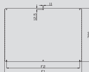
安装板
