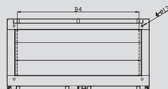
剖面C-C
