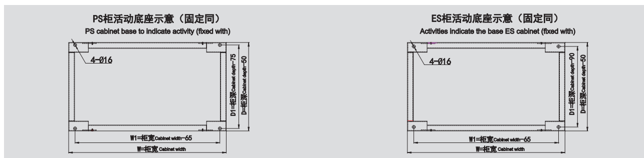
底座开孔图 Base hole diagram
