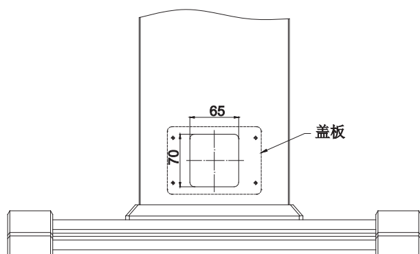
立柱下方背部 A向出线口
