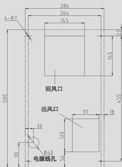
KT450开孔图 KT450 portiforium drawing
