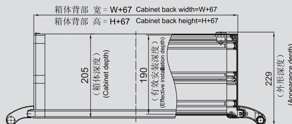
CP190 箱体尺寸 (两侧把手)
