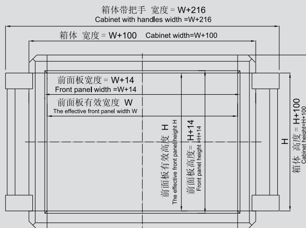
CP190 箱体尺寸 (两侧把手)
