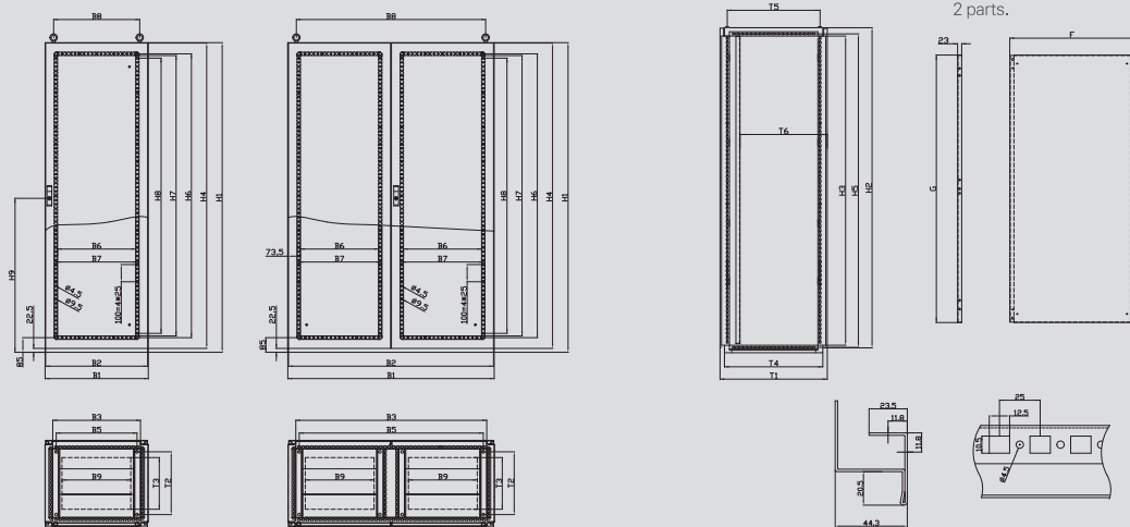
ES/BES 系列细节图 ES/BES Series Detail Drawing
