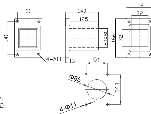
品名: 底座 Part name: support 订货号: 5313800 Order number: 5313800 重量: 5kg Weight: 5kg 材料: 铸钢 Material: cast steel 不可旋转 Not rotatable.
