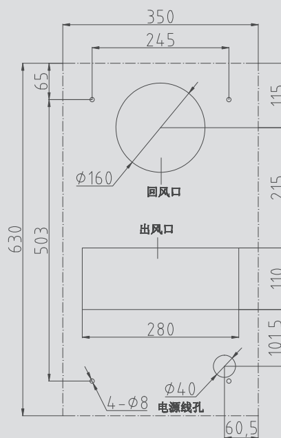
KT800开孔图 KT800 portiforium drawing
