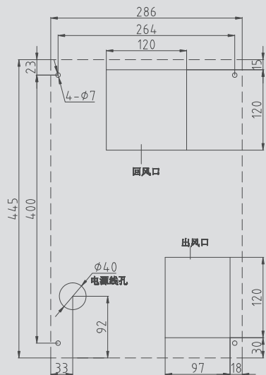
KT300开孔图 KT300 portiforium drawing
