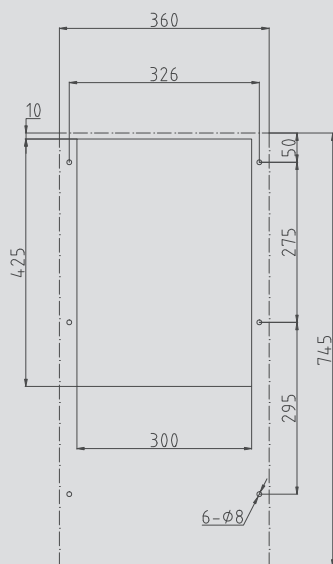
KT1000开孔图 KT1000 portiforium drawing
