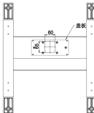
立柱底部 B向出线口
