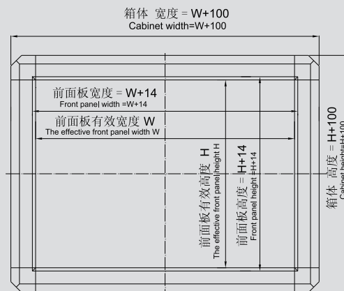
CP140 箱体尺寸 (无把手)
