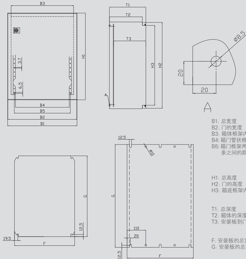
AE/BAE系列细节图 AE/BAE series detail drawing
