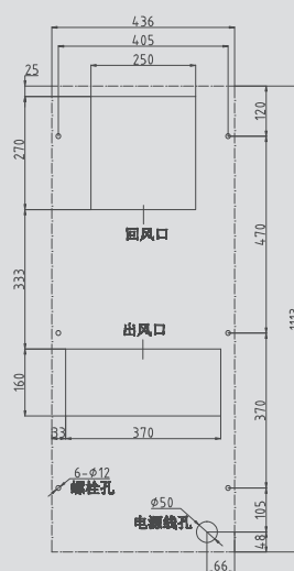
KT2500开孔图 KT2500 portiforium drawing
