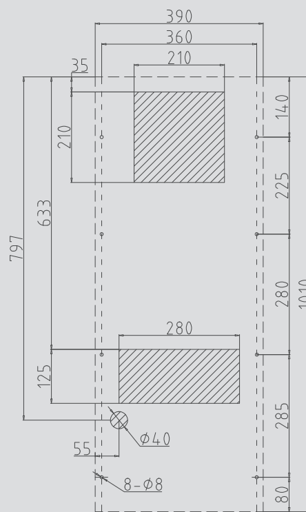
WSKT2000无水空调开孔图 WSKT2000 portiforium drawing
